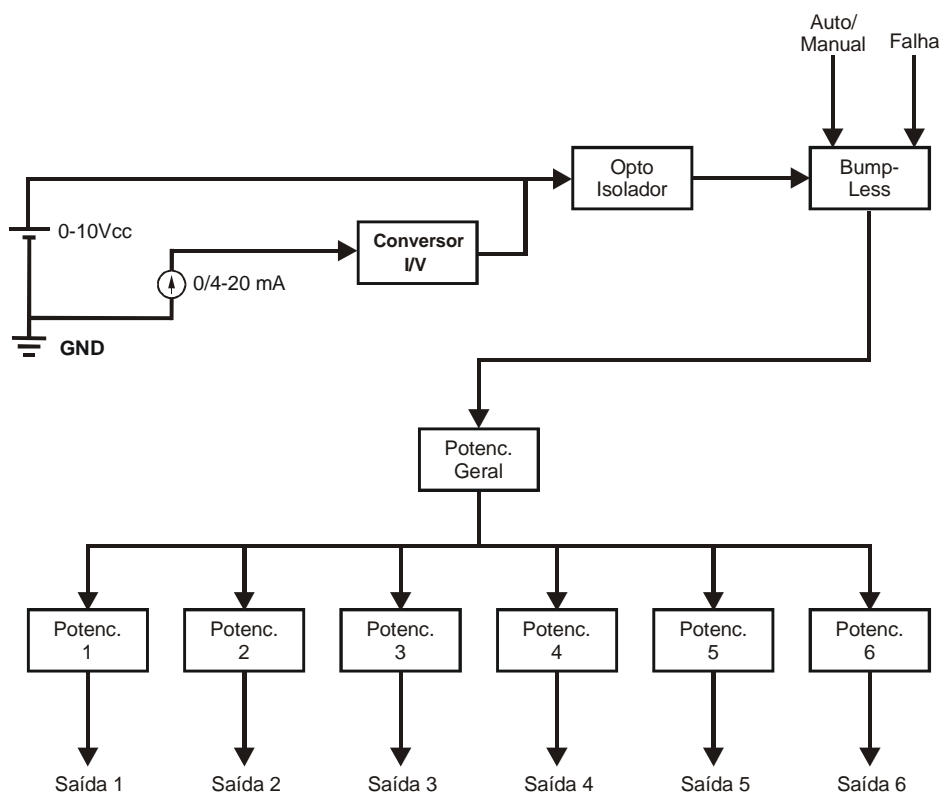
Figura 2 - Diagrama de Blocos Simplificado do WDC-510
