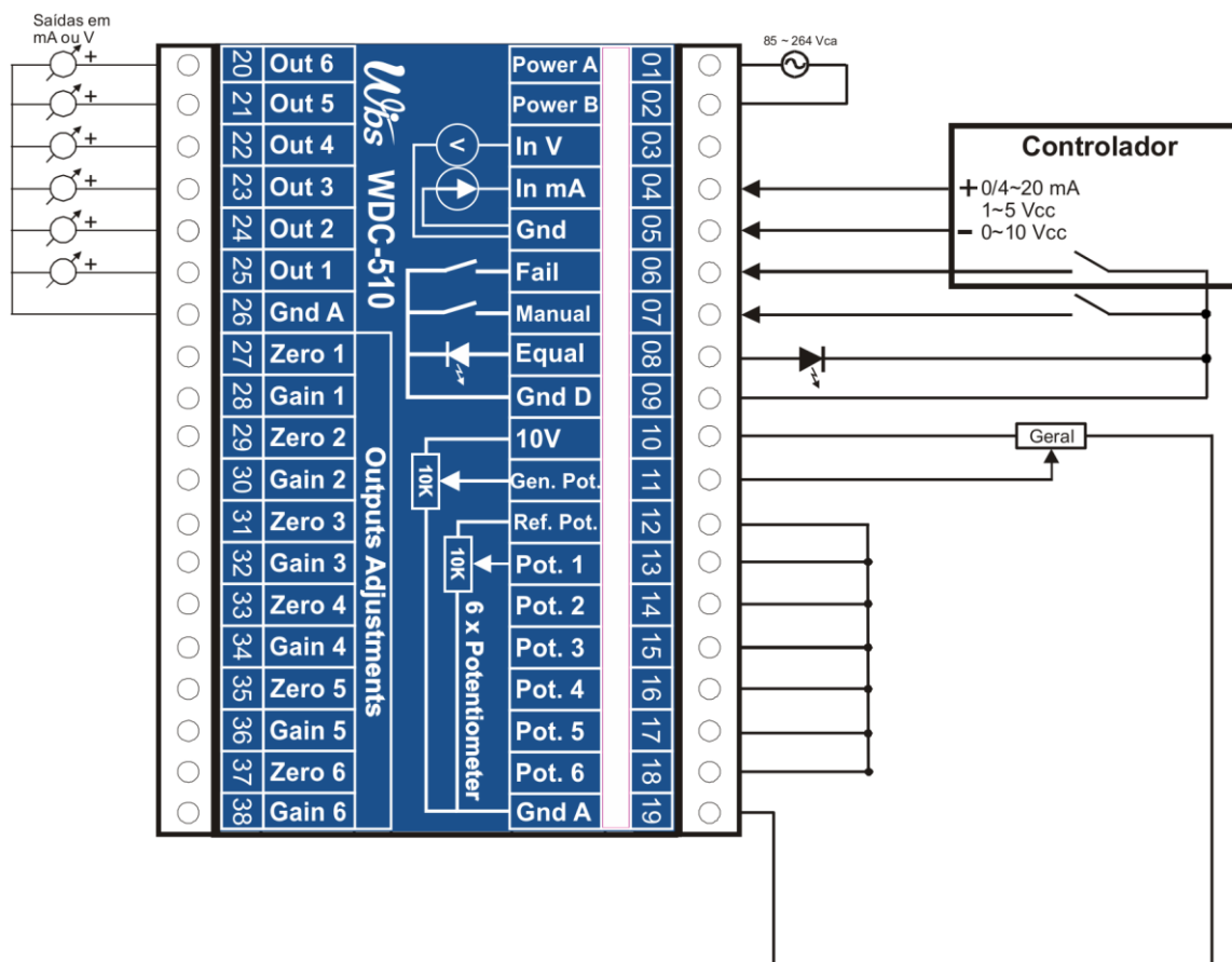
Figura 4 – Esquema de ligação para 1 entrada e 6 saídas, sem o uso de potenciômetros.
