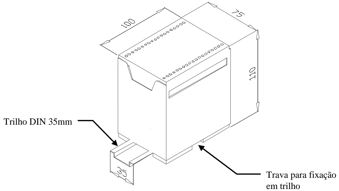
Figura 1 - Dimensões (em mm) do WDC-510
