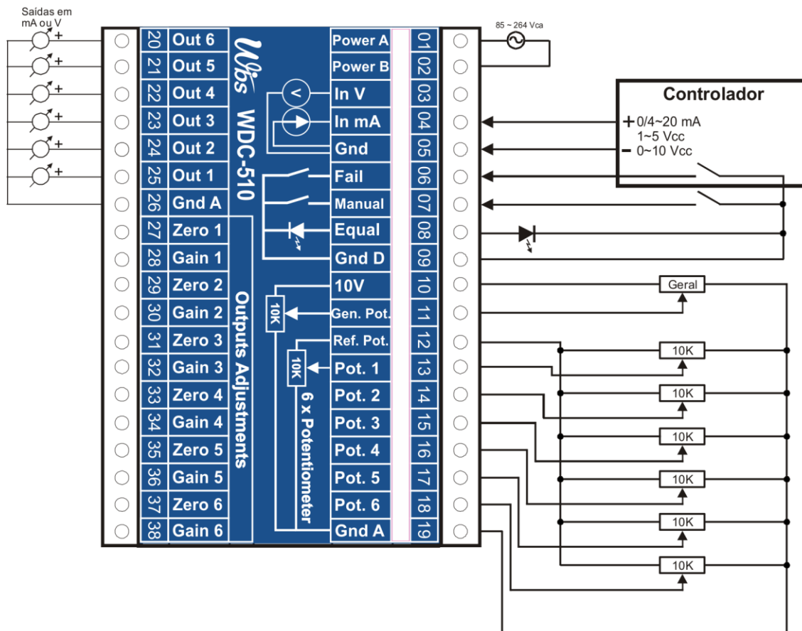
Figura 3 - Esquema de ligação para 1 entrada e 6 saídas, com potenciômetros
