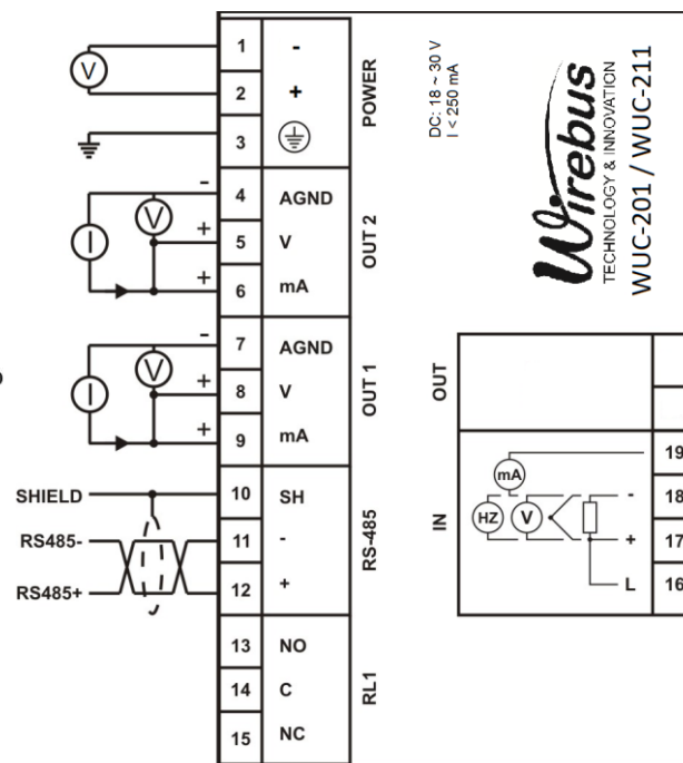
Figura 5 – Borneias (DC)
