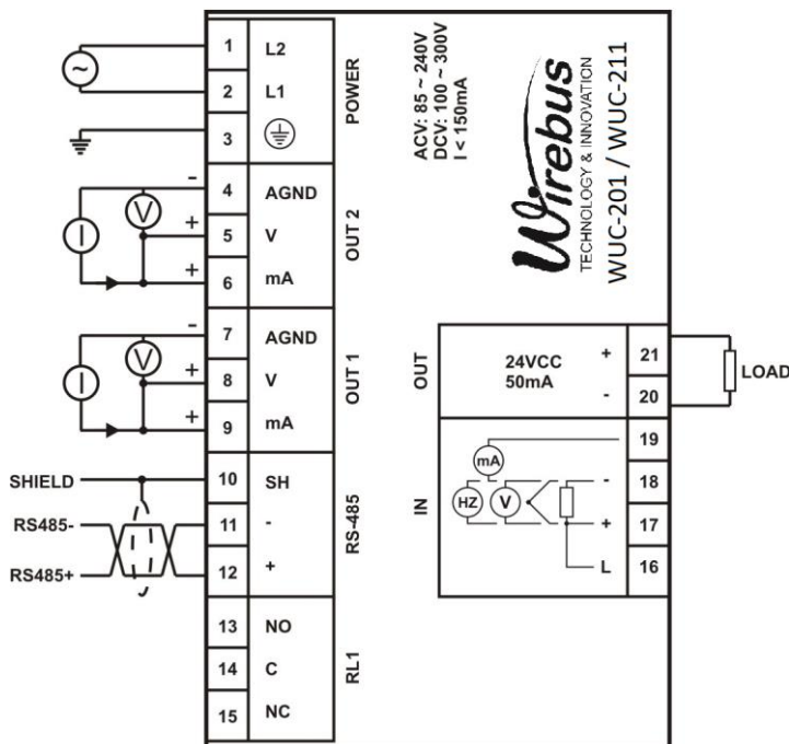
Figura 3 – Borneias (AC)
