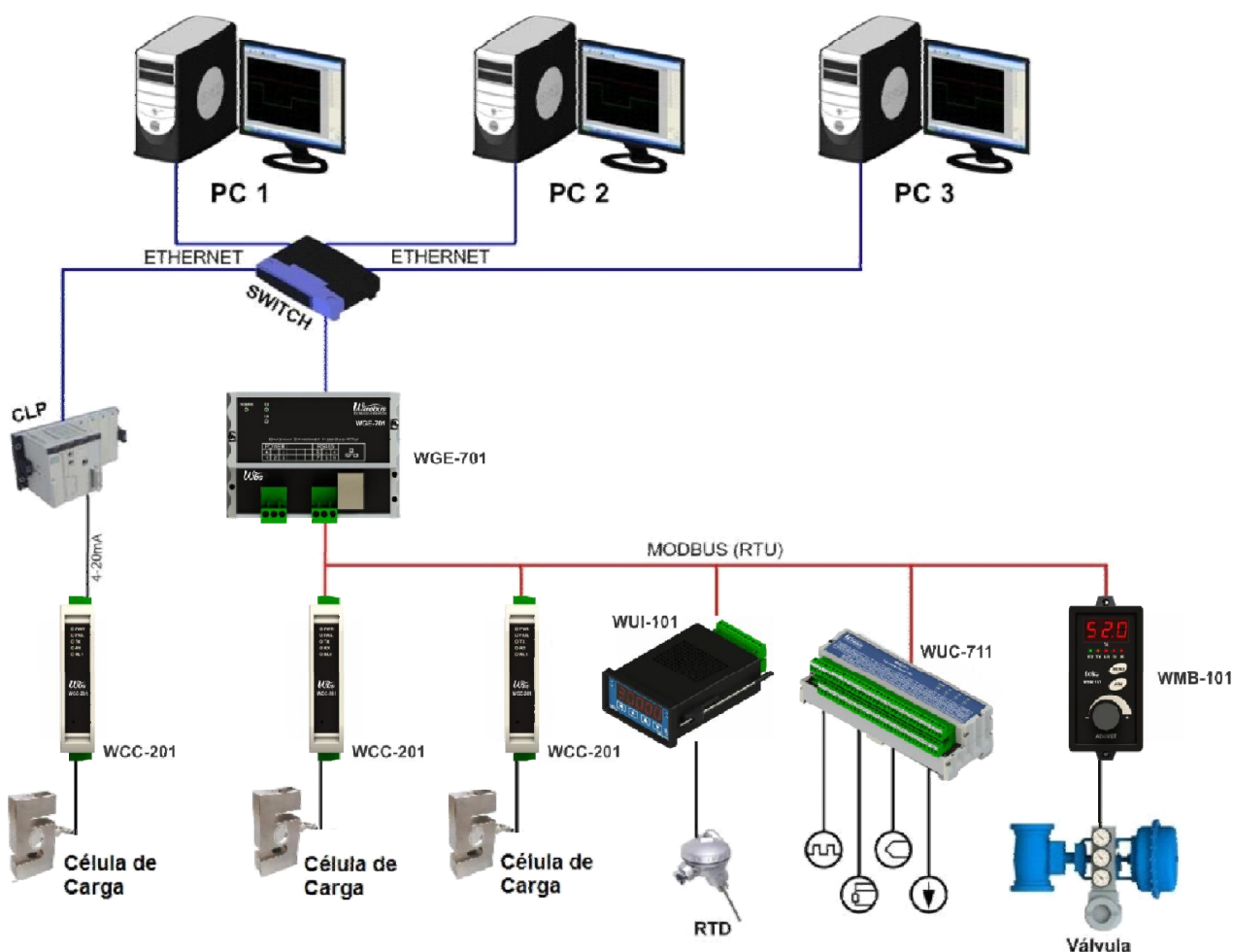
Figura 2 – Topologia rede Modbus com a WCC-201
